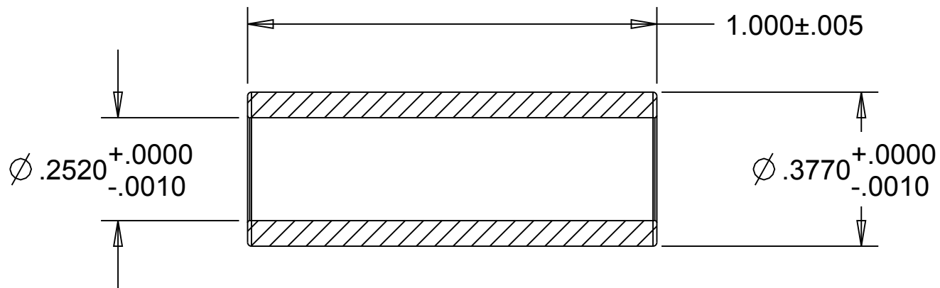
SECTION A-A
