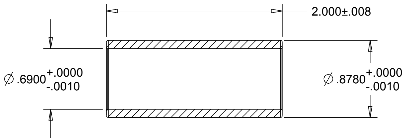
SECTION A-A
