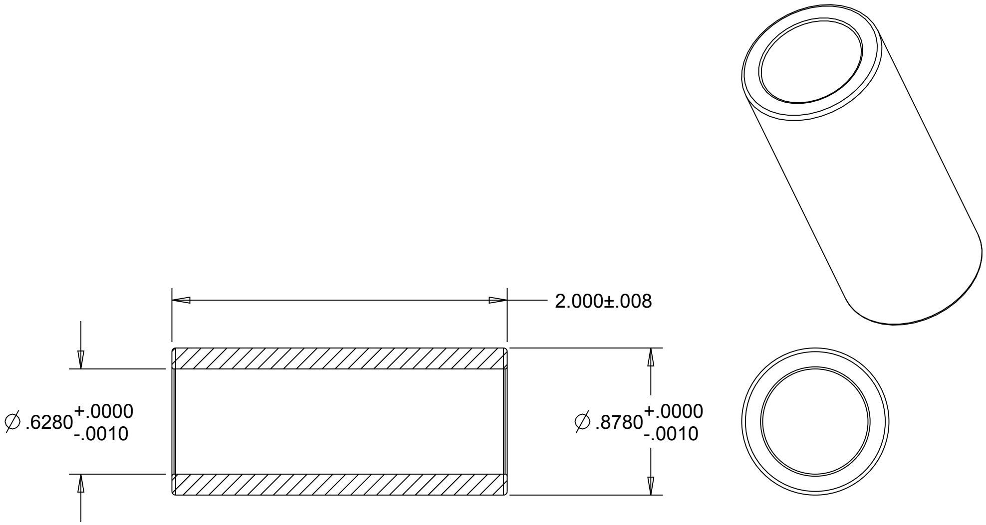
SECTION A-A
