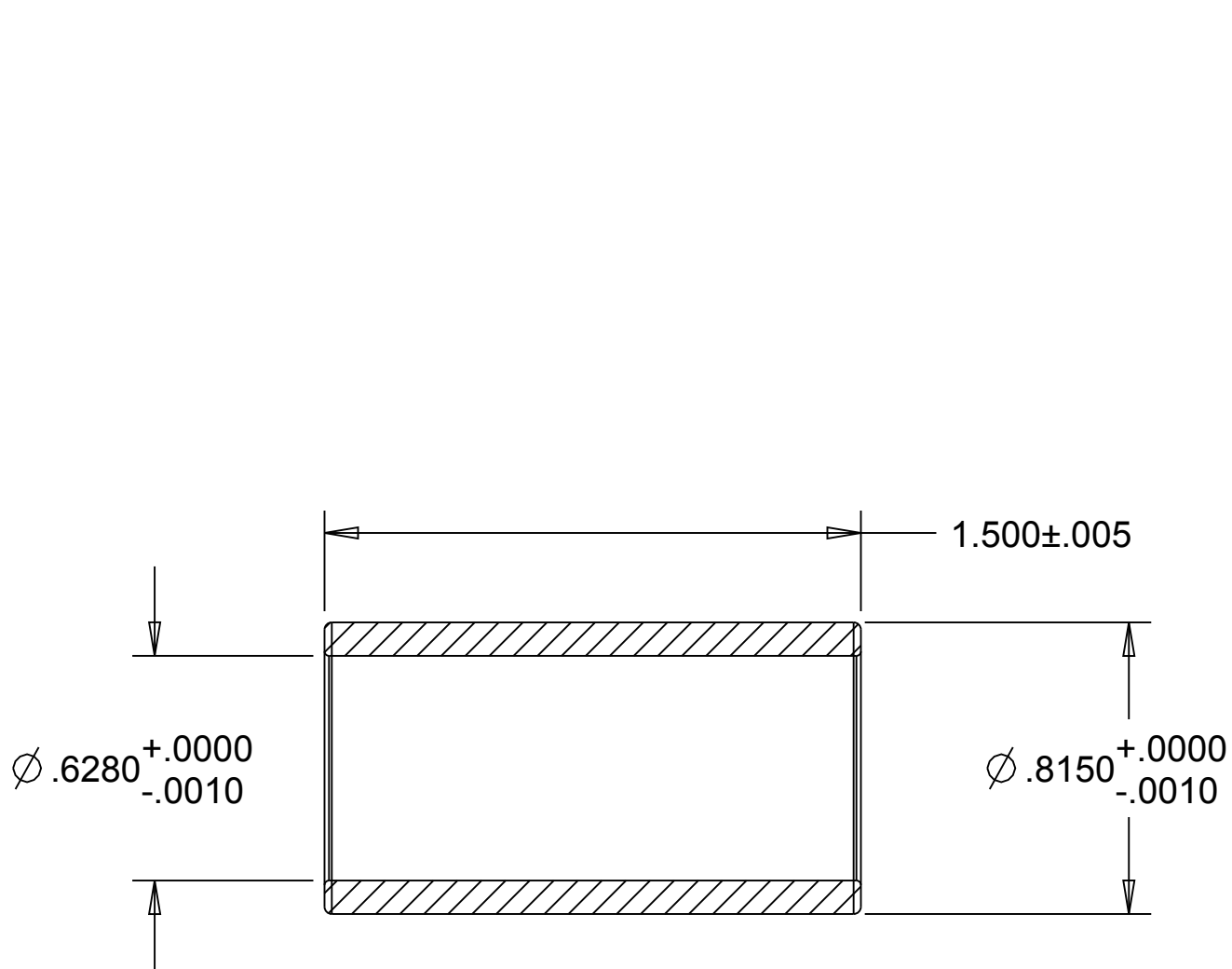
SECTION A-A
