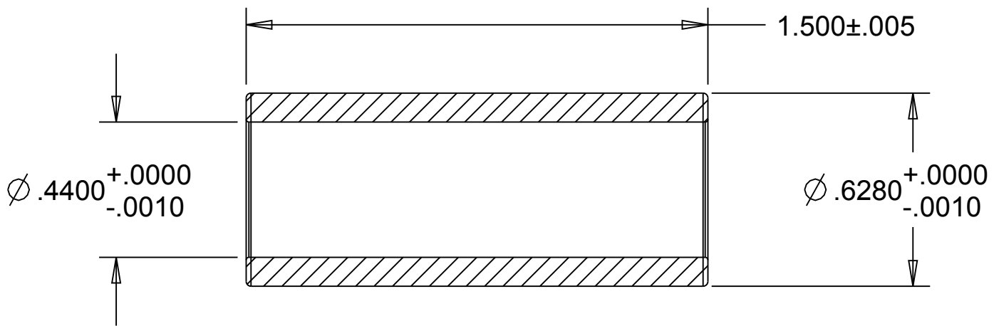
SECTION A-A
