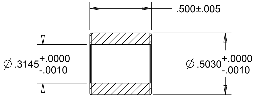
SECTION A-A
