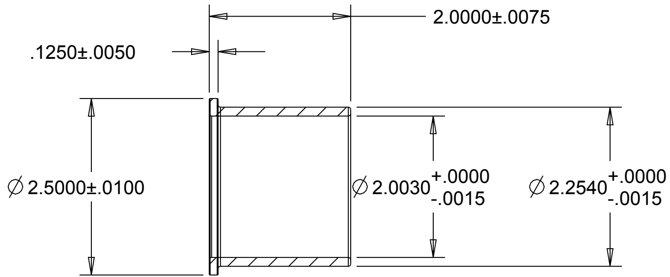
SECTION A-A
