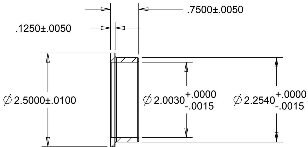
SECTION A-A
