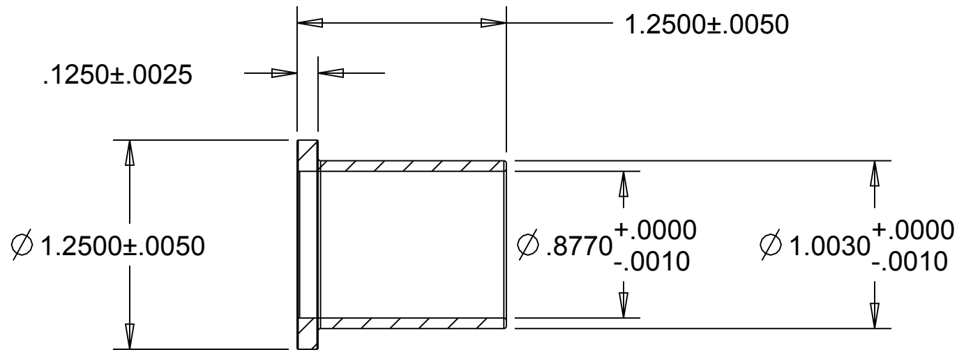
SECTION A-A
