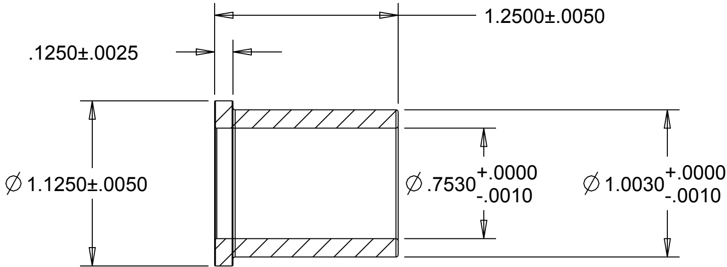
SECTION A-A
