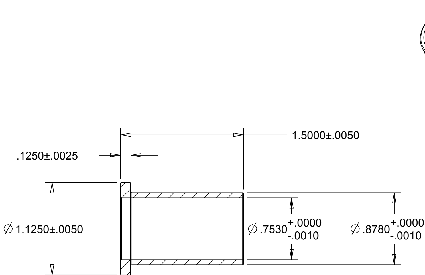
SECTION A-A
