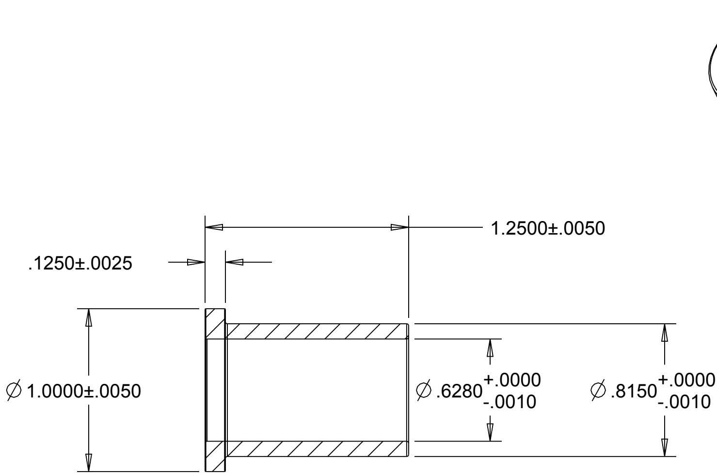
SECTION A-A
