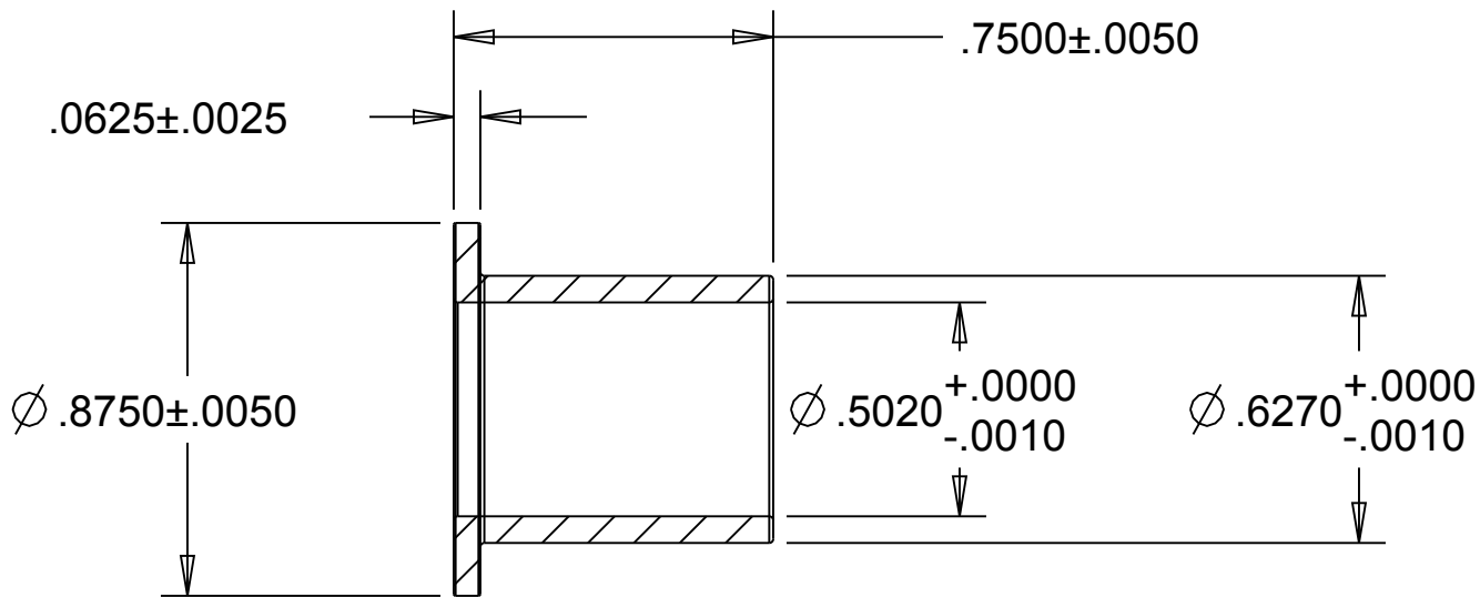
SECTION A-A
