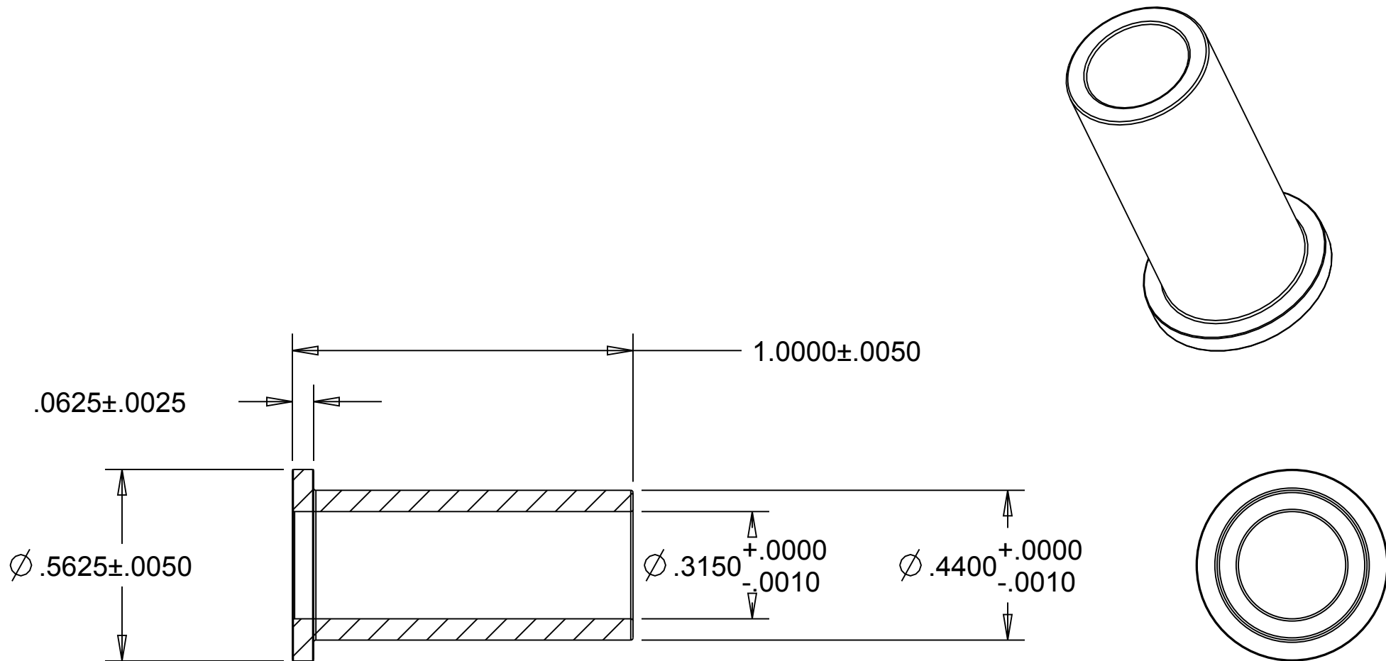
SECTION A-A
