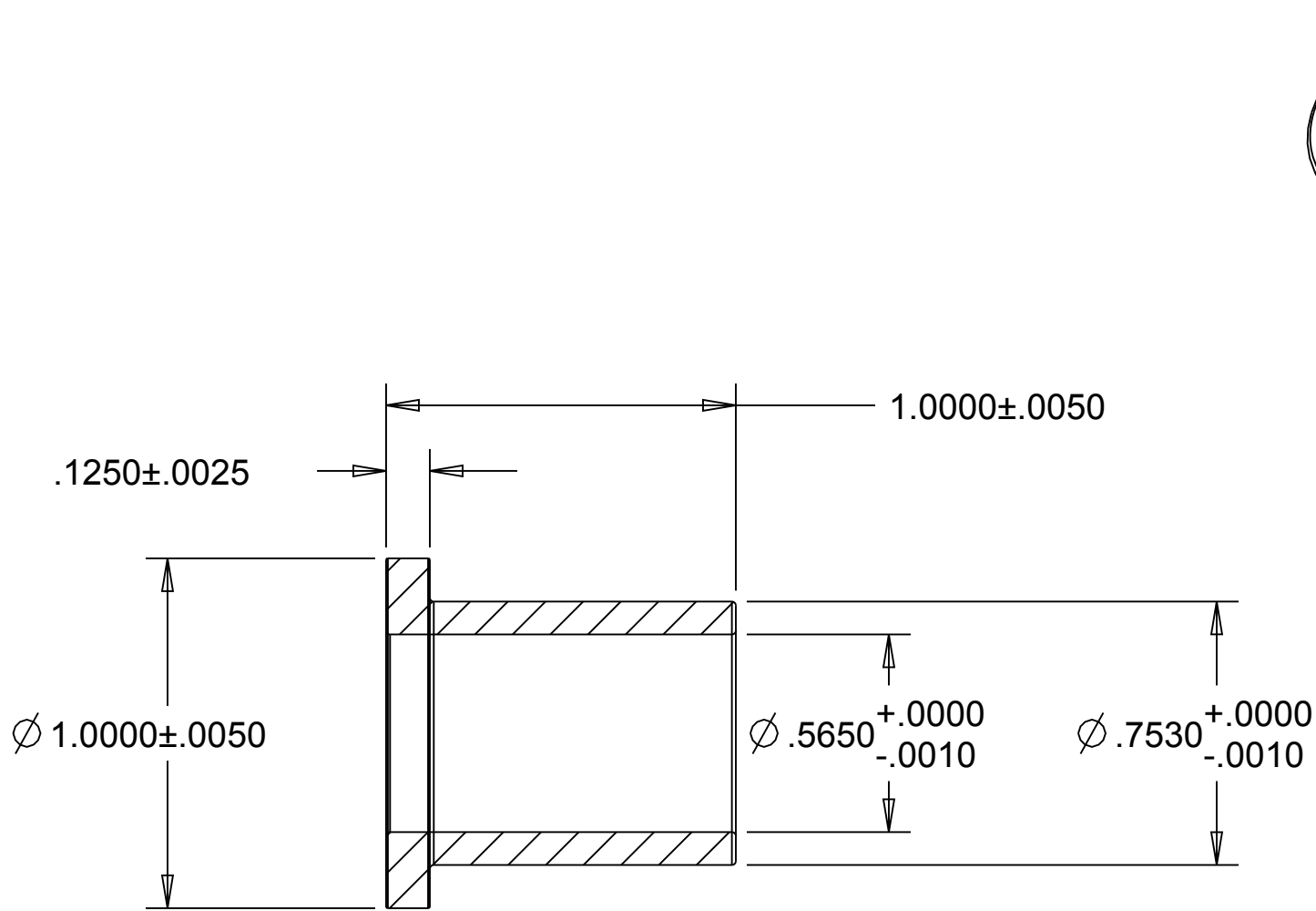
SECTION A-A
