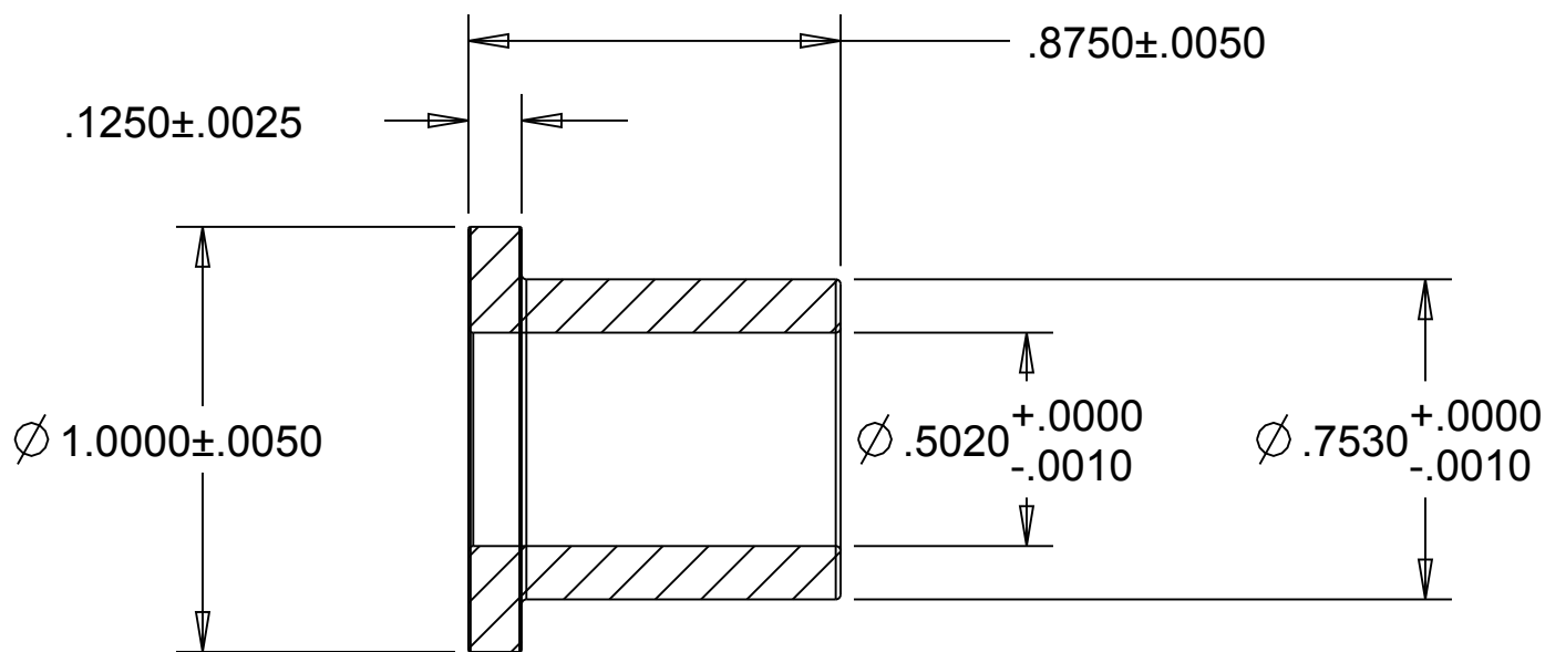
SECTION A-A
