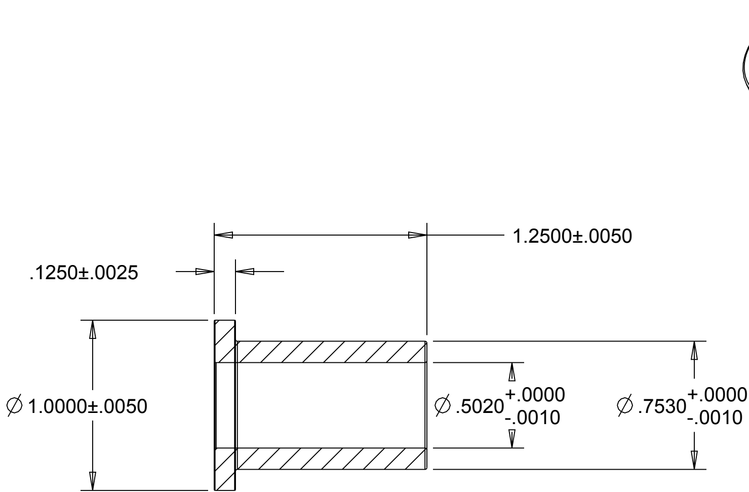
SECTION A-A
