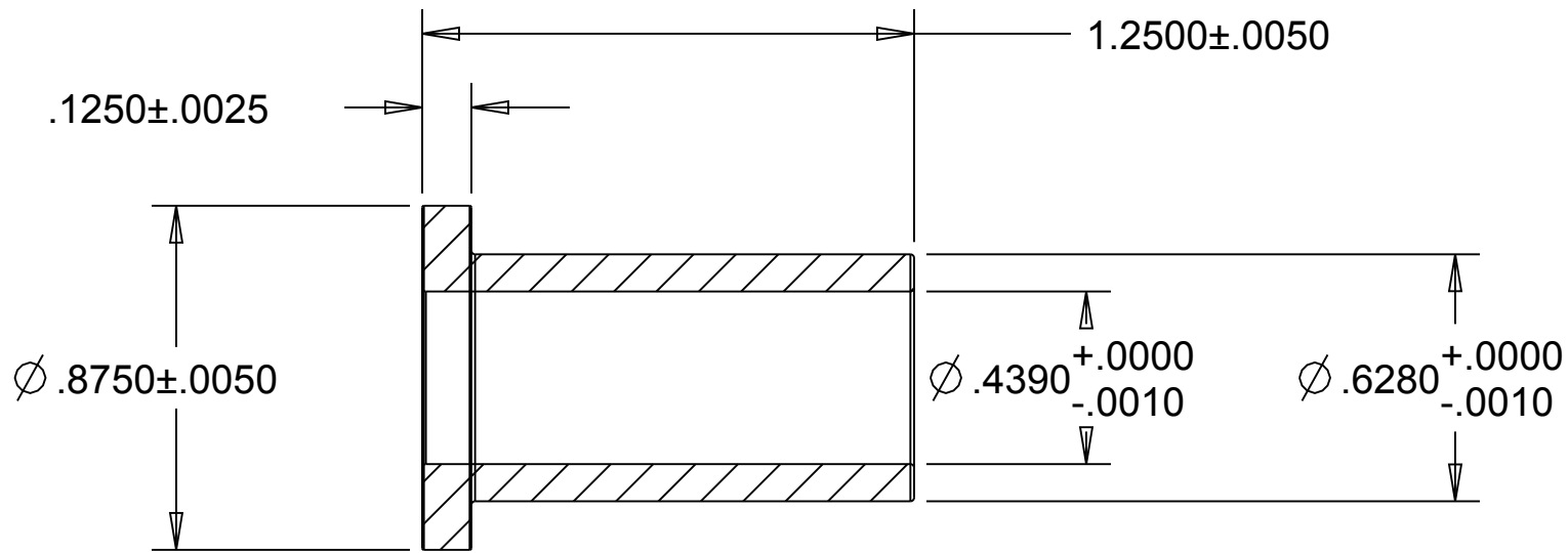
SECTION A-A
