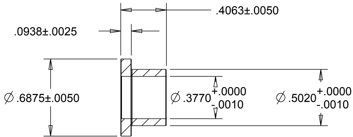
SECTION A-A
