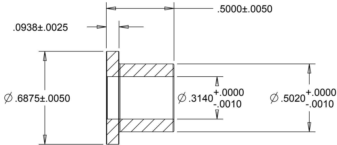
SECTION A-A
