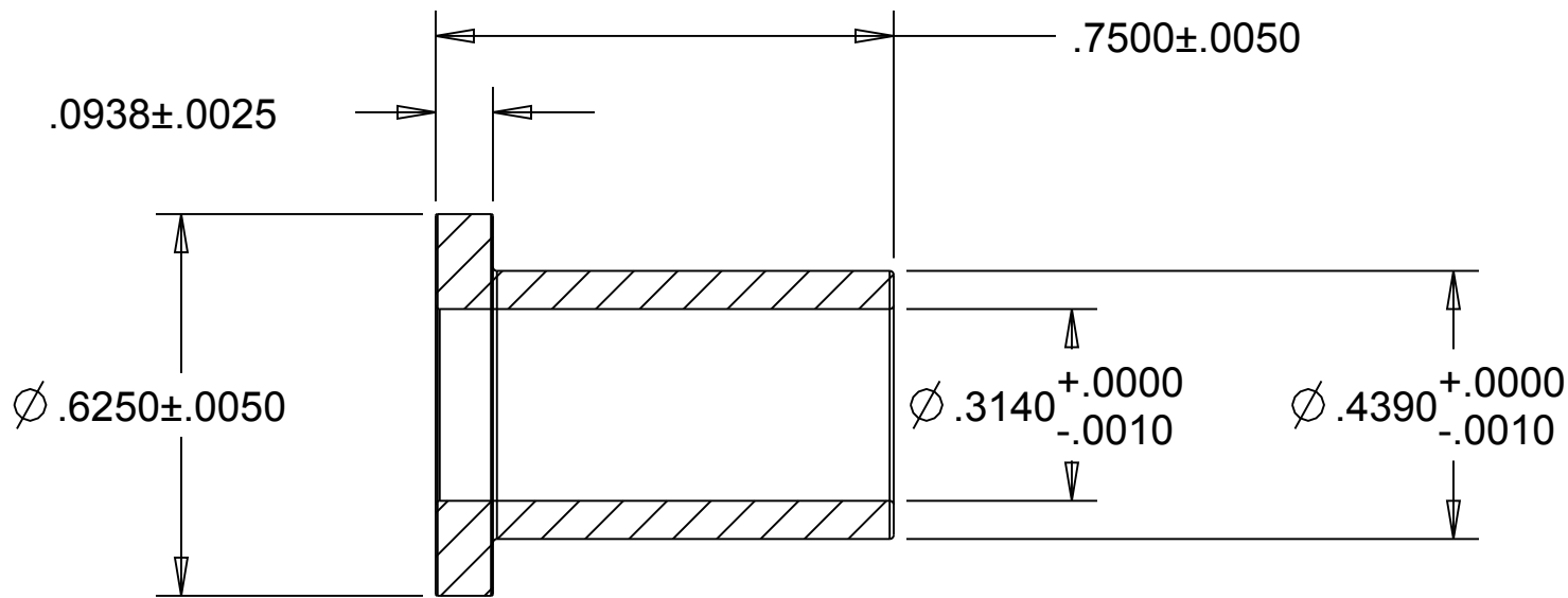
SECTION A-A
