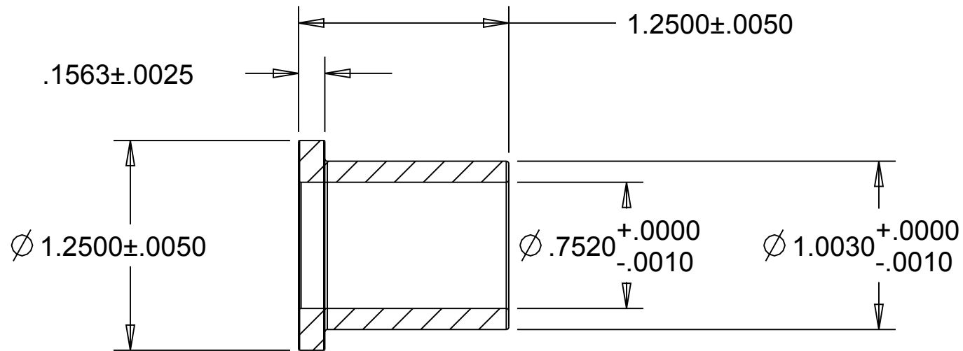
SECTION A-A
