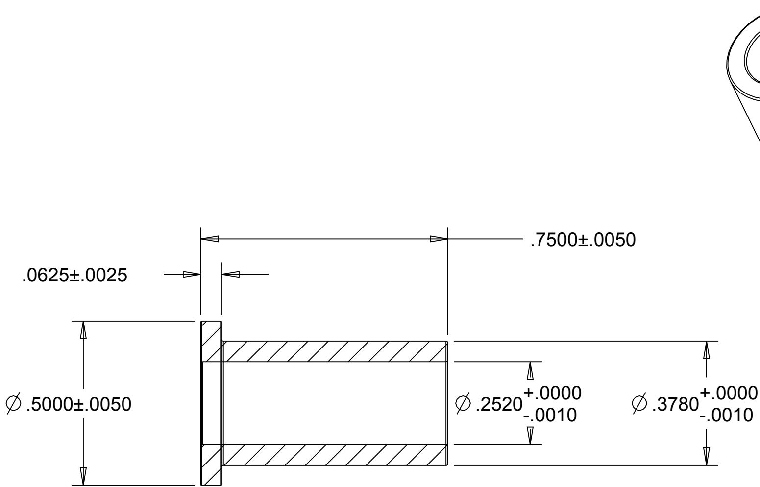
SECTION A-A
