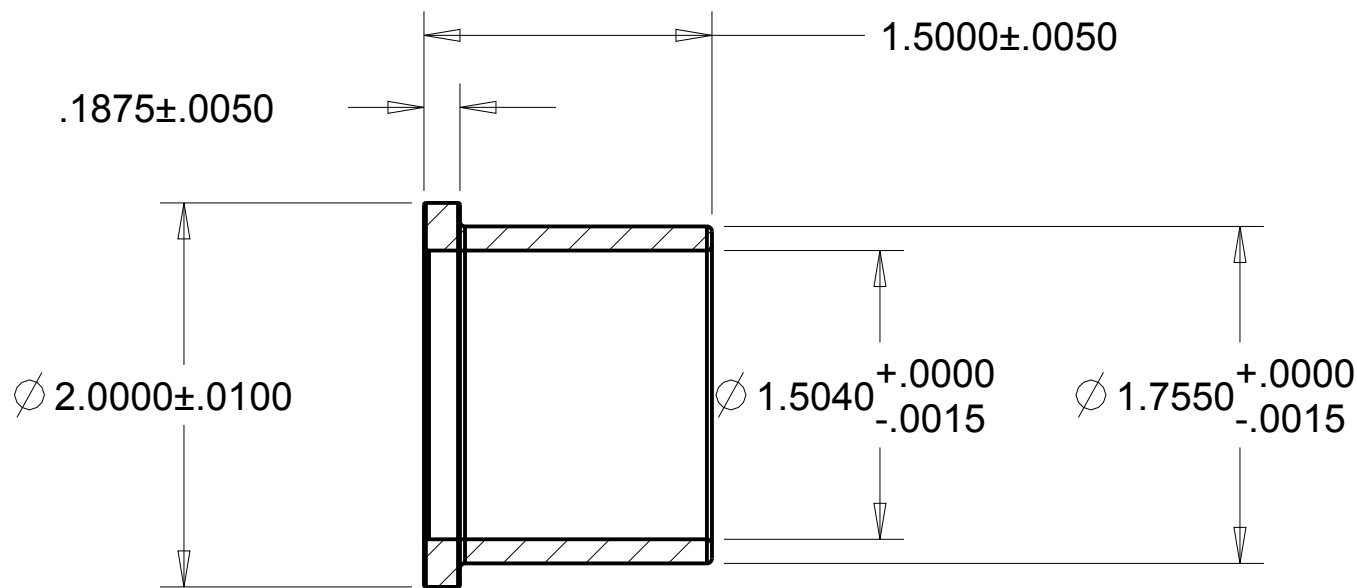
SECTION A-A
