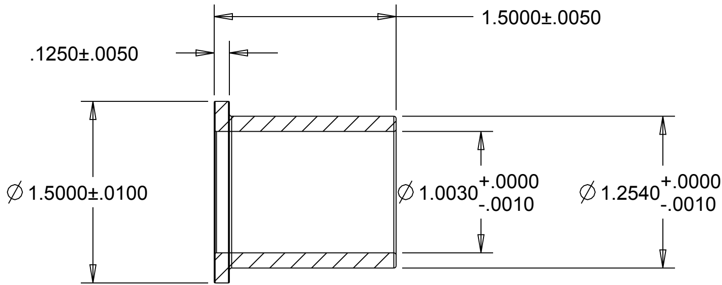
SECTION A-A
